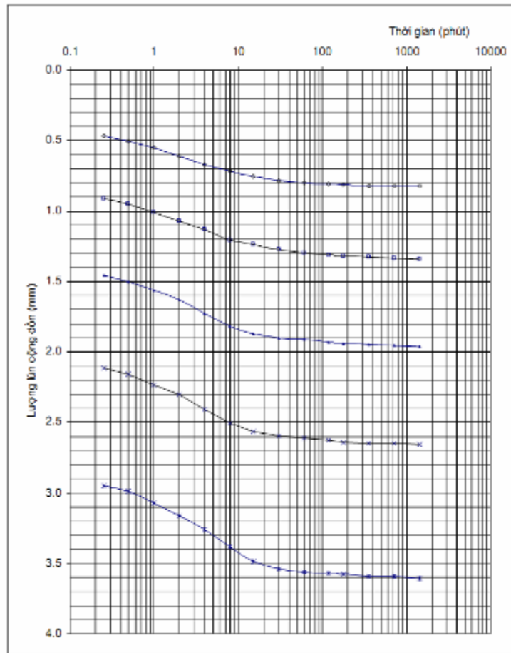
Hình C.3- Lượng lún cộng dồn
