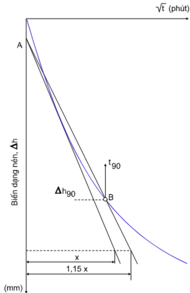
Hình 1 - Đường cong cố kết.
