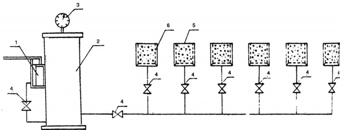
Hình 1 – 1. Bơm ; 2. Thùng dâng áp ; 3. Đồng hồ áp lực ; 4. Van chịu áp lực ; 5. Mẫu thử ; 6. Áo mẫu.
